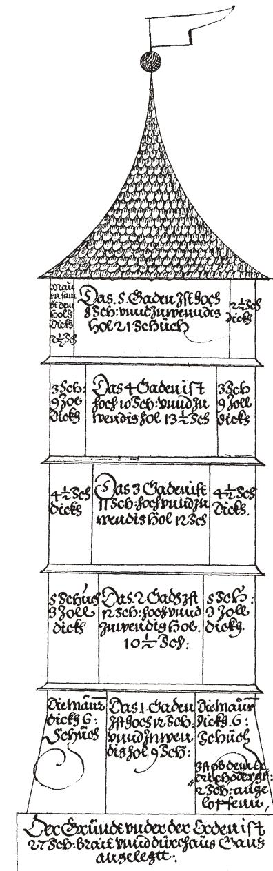
Mit Maßangaben versehene Aufrisszeichnung für den Michelsturm, der nach seinem Einsturz mit dickeren Mauern wieder aufgebaut werden sollte (Gaden ist die alte Bezeichnung für Stockwerk)
